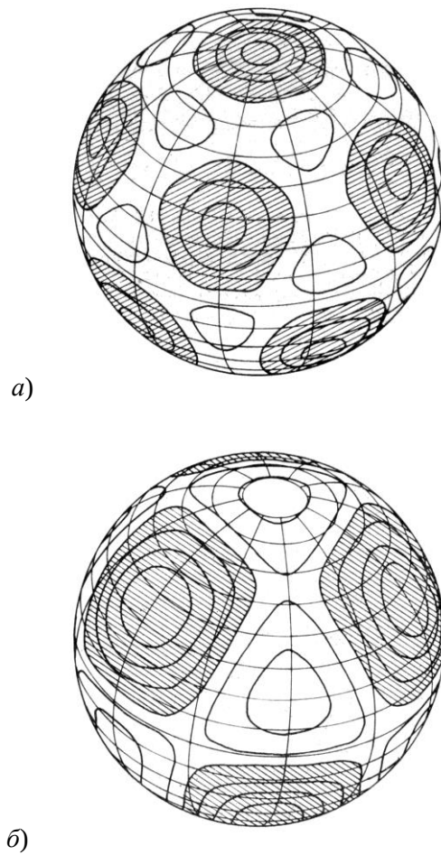
Рис. 3.2. Конвекция в пограничном сферическом слое по Буссе (1975): а) при образовании в каждой полусфере 6-и главных геометрических фигур – пятиугольников и 10 промежуточных фигур – треугольников; б) при образовании в каждой полусфере 3-х главных фигур – квадратов и 4-х промежуточных фигур – треугольников
