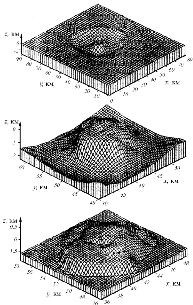
Рис. 4.5. Рельеф поверхности истинного дна Пучеж-Катунской импактной структуры: a – астроблемы в целом; б – центрального поднятия; в – свода центрального поднятия выше изогипсы 0,5 км. Соотношение вертикального и горизонтального масштабов 1: 3
