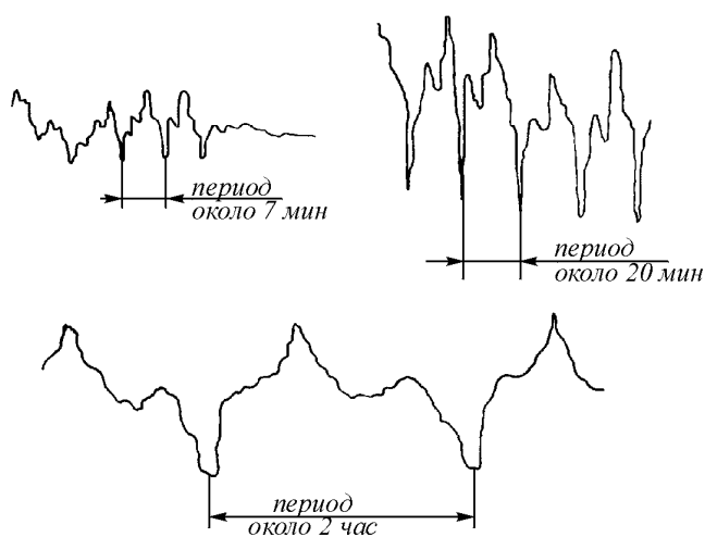
Рис. 3.4. Типовые вариации эфирного ветра, обнаруженные при измерениях отклонений лазерного луча (бывают вариации и со значительно более короткими периодами)
