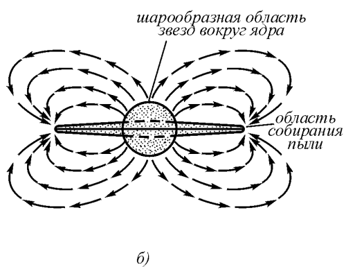
Рис. 2.9. Структура спиральной галактики: а – вид на плоскость; б – вид сбоку
