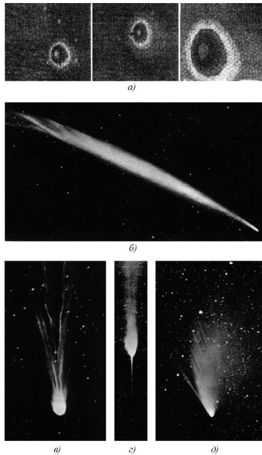
Рис. 4.3. Фотографии комет: а – комета Хиякутаки, 1996 г., отчетливо видна тороидальная структура; б – комета Икея–Секи, 1965 г., у кометы веретенообразный задний «хвост»; в – комета Икея, 1963 г., задний «хвост» расширен и расщеплен; г – комета Аренда–Ролана, 1957г., у кометы появился передний острый «хвост»; д – комета Маркоса, 1957 г., вещество рассеивается, комета близка к гибели
