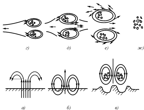
Рис. 4.2. Образование кометы: а) начальный этап; б) формирование в) выход кометы в космос; г) образование заднего «хвоста»; д) образование переднего «хвоста»; е) разброс вещества; ж) метеорный поток, оставшийся после кометы
