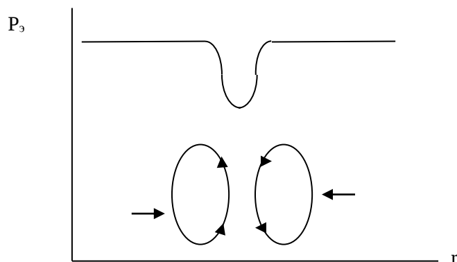
Рис. 2.3. Сущность сильного ядерного взаимодействия
